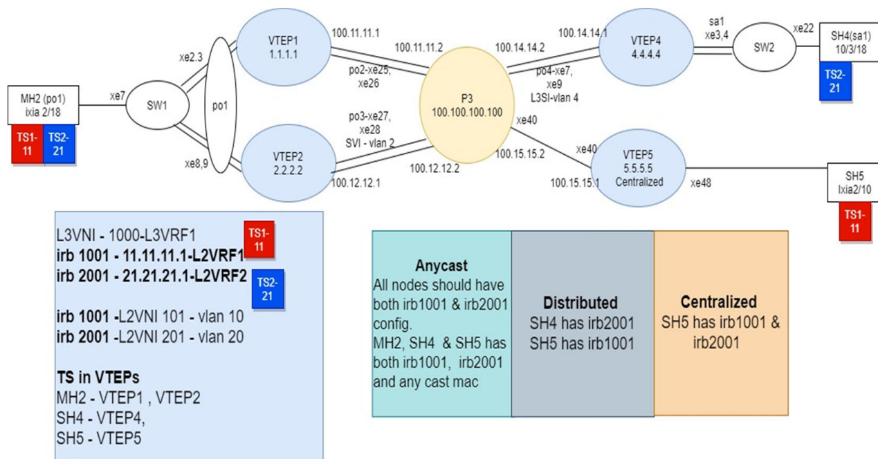
Figure 1-8: VxLAN EVPN IRB
